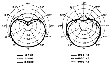
典型的极坐标图形 图 3
